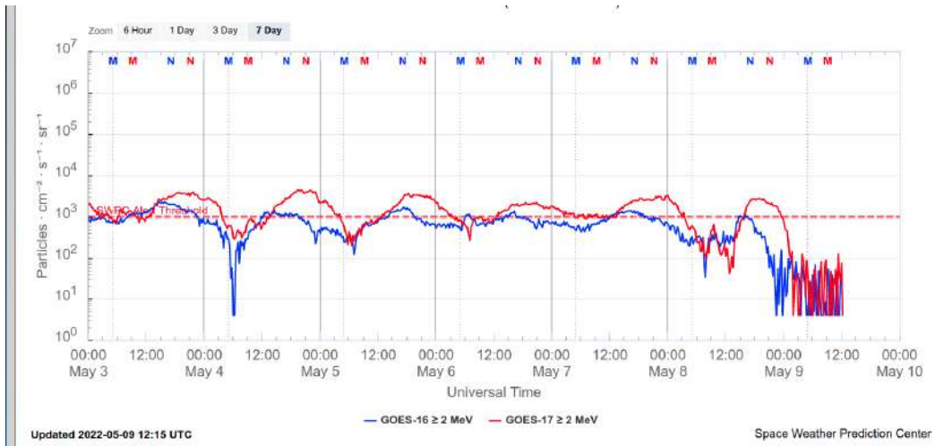
Figura 1: Fluxo de elétrons de alta energia ( \geq 2\text{MeV} ) obtido a partir dos satélites GOES-16 e GOES-17. Fonte
