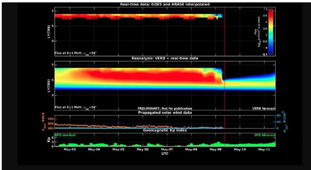
Figura 2: Dados de fluxo de elétrons de alta energia (reais e interpolados) obtidos a partir dos satélites ARASE, GOES-16, GOES-17. Dados reanalisados a partir do VERB code e do fluxo de elétrons interpolados. Dados da velocidade do vento solar e densidade de prótons obtidos a partir do satélite ACE. Fonte
