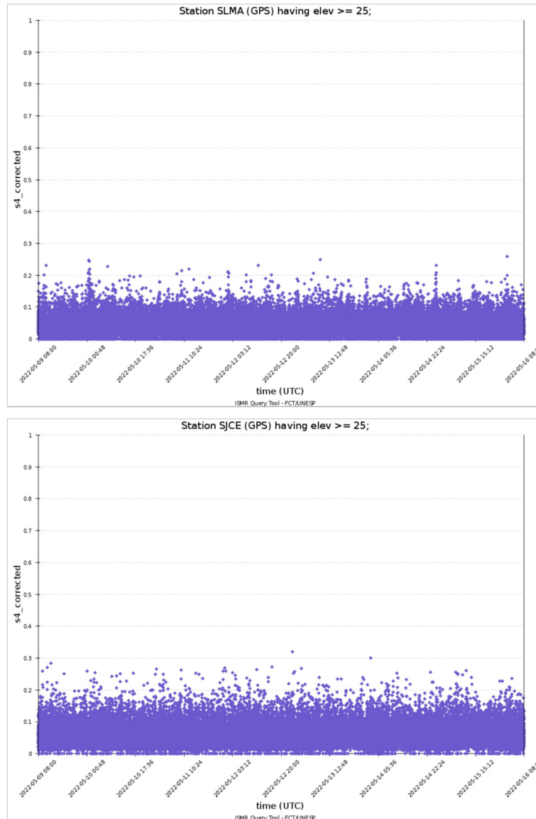
Figura 1: Valores do índice S4 para a constelação GPS para a estação SLMA (painel superior) e a estação SJCE (painel inferior) durante a semana 9—16/05 .
