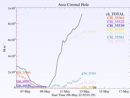
Figura: A linha em preto mostra o resultado da soma das áreas para cada intervalo da detecção realizado pelo SPOCA entre os dias 06 e 13 de maio de 2022
